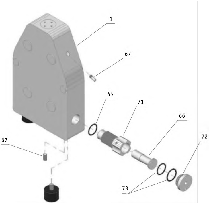
Пневматическая система обратного слива
