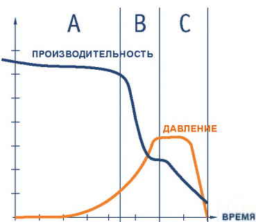
ТИПИЧНЫЙ РАБОЧИЙ РЕЖИМ ФИЛЬТР-ПРЕССА
