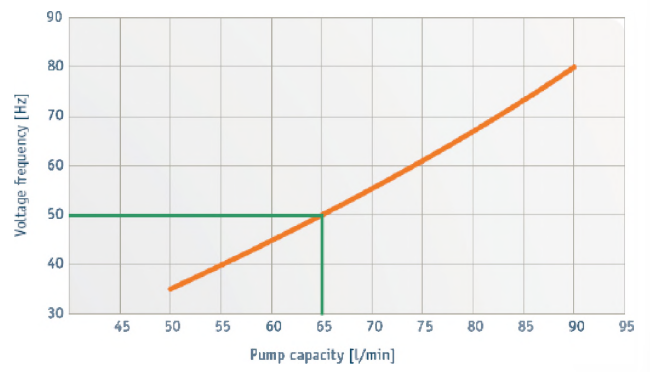
DME 25
