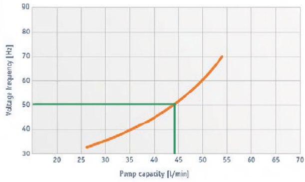
DME 40 R(Z)..
