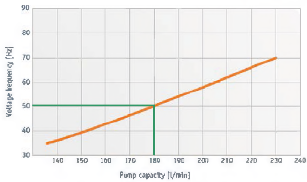
DME 40 R(Z)..
