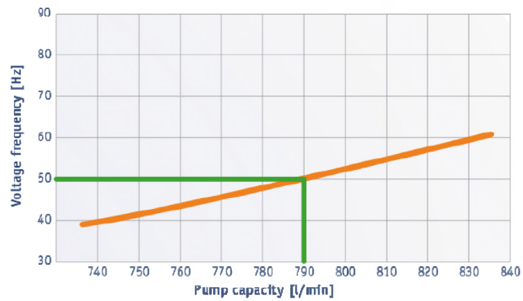
DME 80
