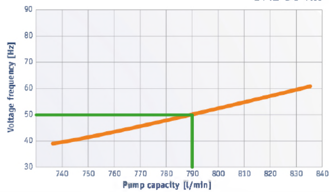
DME 80 R..
