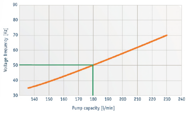
DME 40
