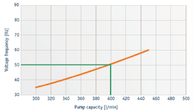
DME 80 R..
